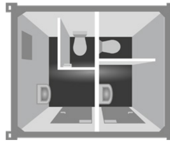
WC-CONTAINER 10 FT
